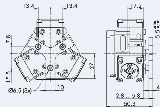
卸料器外形尺寸 卸料器行程 3 mm 最小弹簧力 18N
