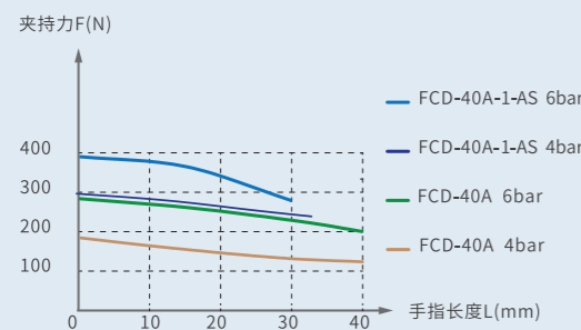
外夹抓取
