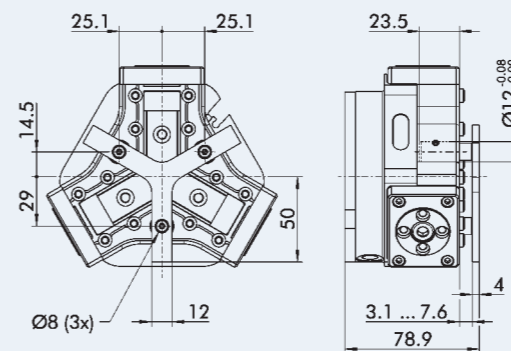
卸料器外形尺寸 卸料器行程 4.5 mm 最小弹簧力 35N
