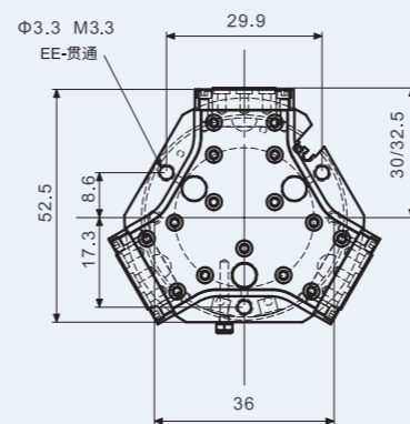
卸料器外形尺寸 卸料器行程 2.6 mm 最小弹簧力 11N
