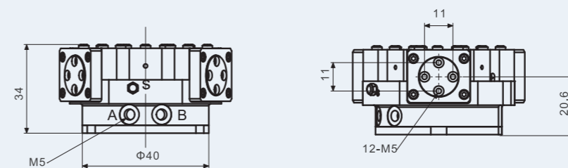
1 常规款尺寸图
