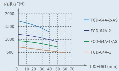
内撑抓取
