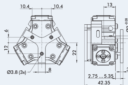
卸料器外形尺寸 卸料器行程 2.6 mm 最小弹簧力 11N
