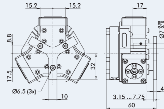
卸料器外形尺寸 卸料器行程 4.6 mm 最小弹簧力 11N
