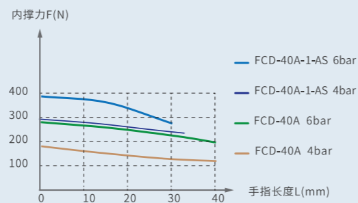
内撑抓取
