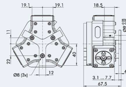
卸料器外形尺寸 卸料器行程 4.6 mm 最小弹簧力 18N
