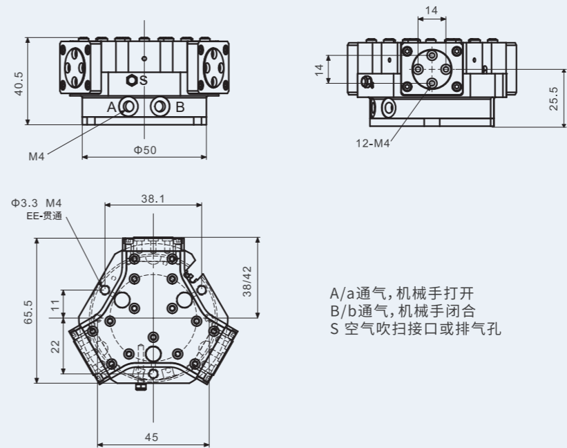
卸料器外形尺寸 卸料器行程 3 mm 最小弹簧力 18N
